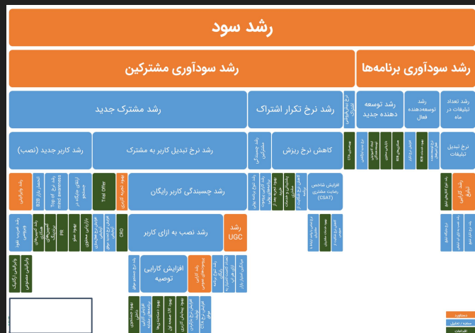
درخت KPI
